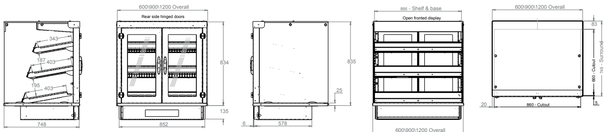
End Elevation
