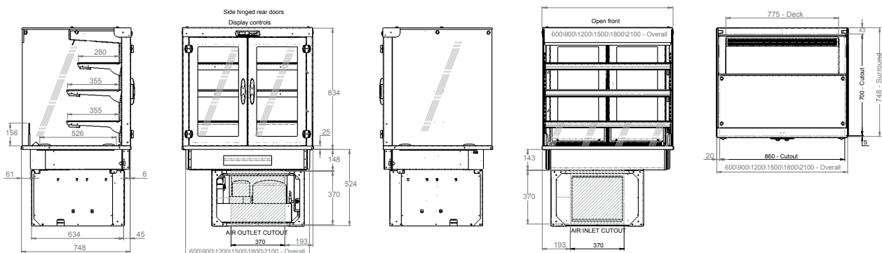
End Elevation
