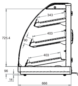
End Elevation
