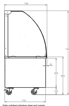
End Elevation
