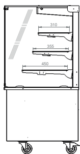
End Elevation
