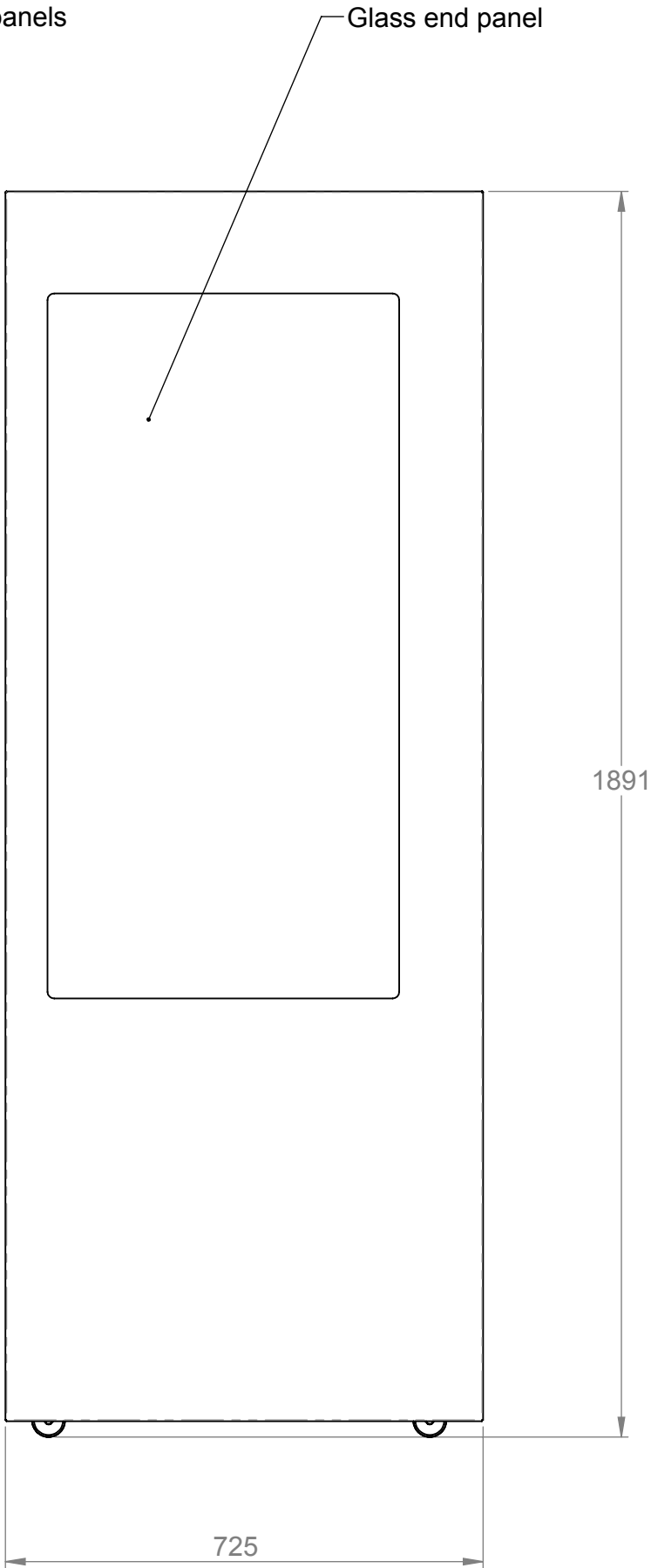
End elevation
