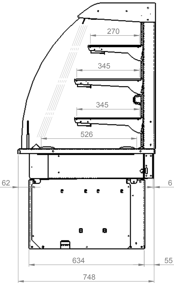
End elevation
