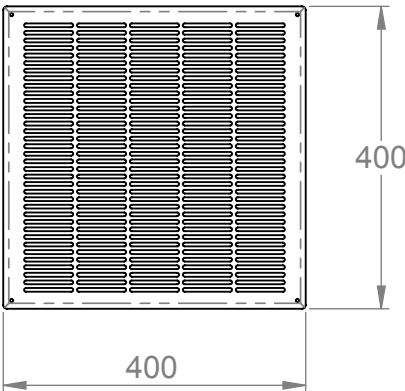
End elevation
