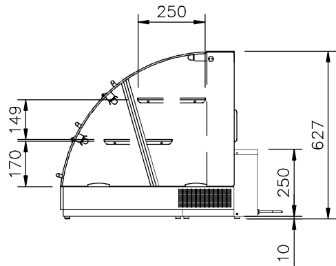
END ELEVATION
