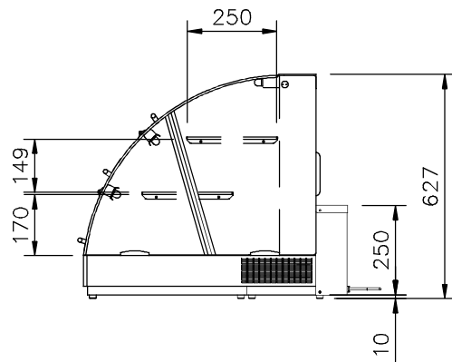
END ELEVATION
