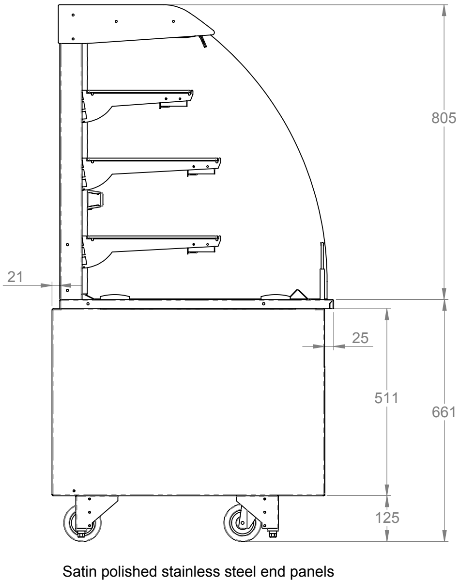
End elevation
