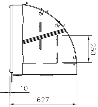
END ELEVATION
