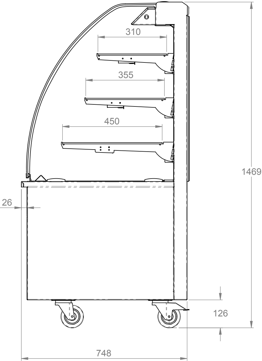
End elevation
