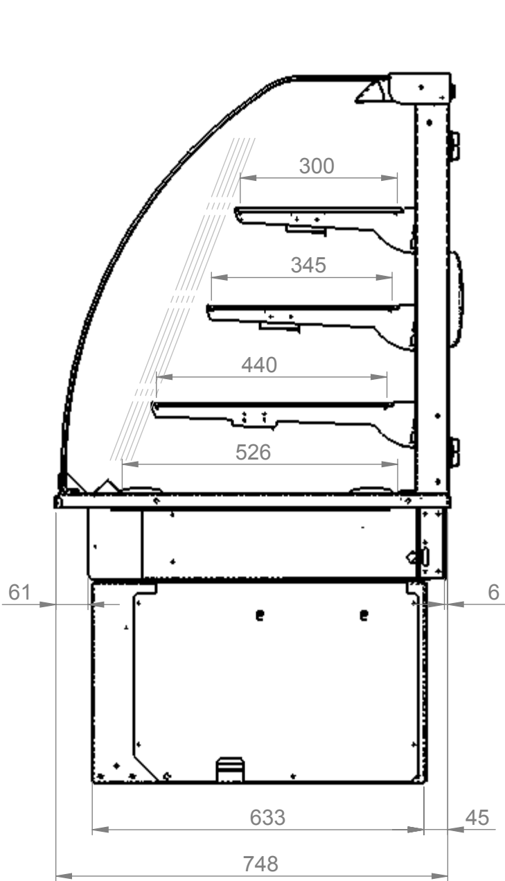
End elevation
