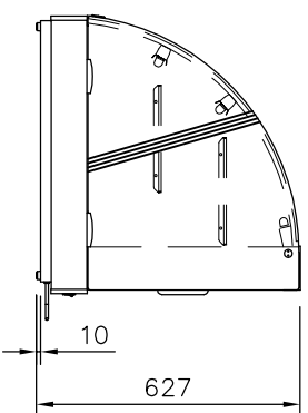
END ELEVATION
