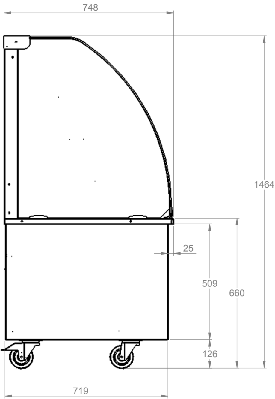
End elevation
