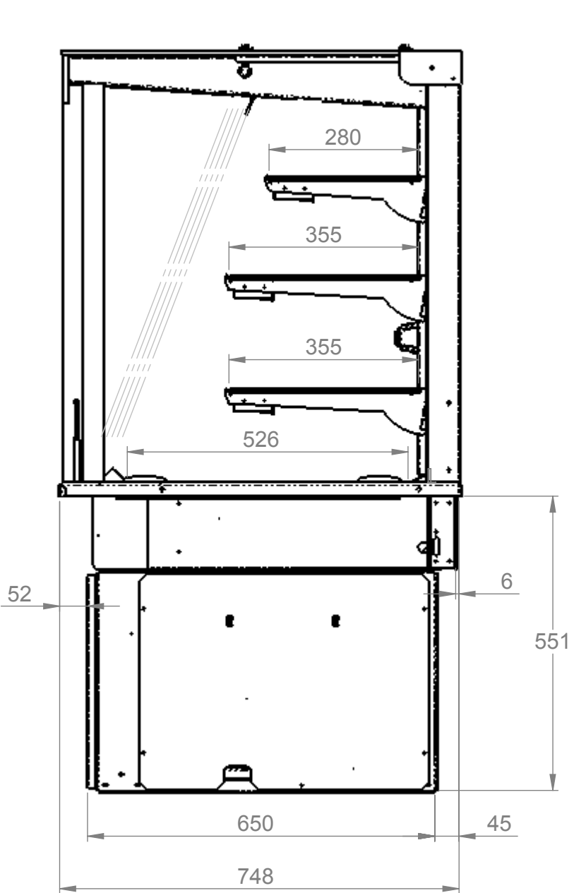
End elevation
