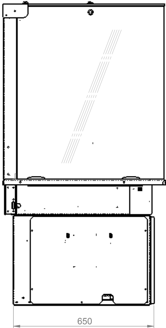
End elevation
