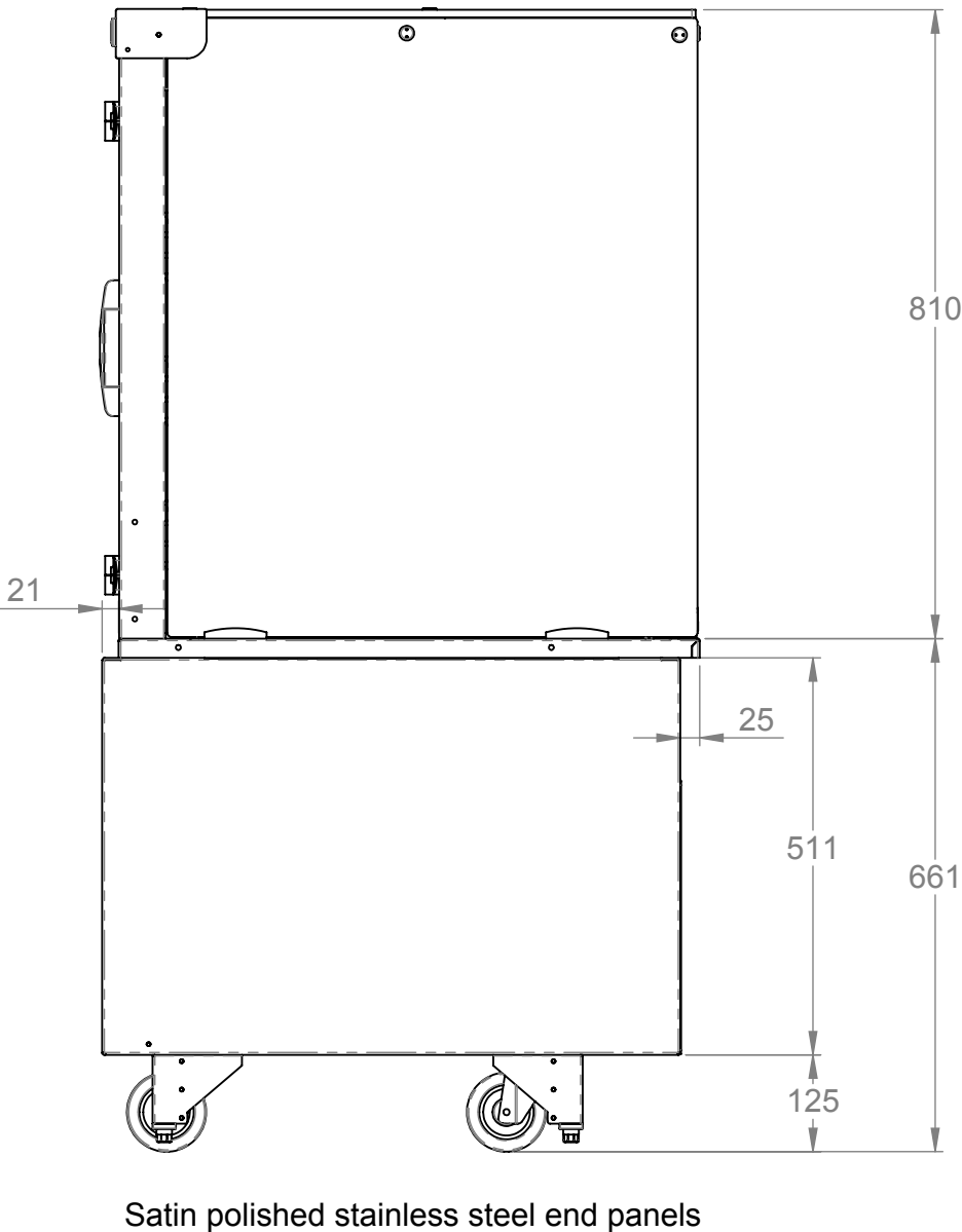
End elevation
