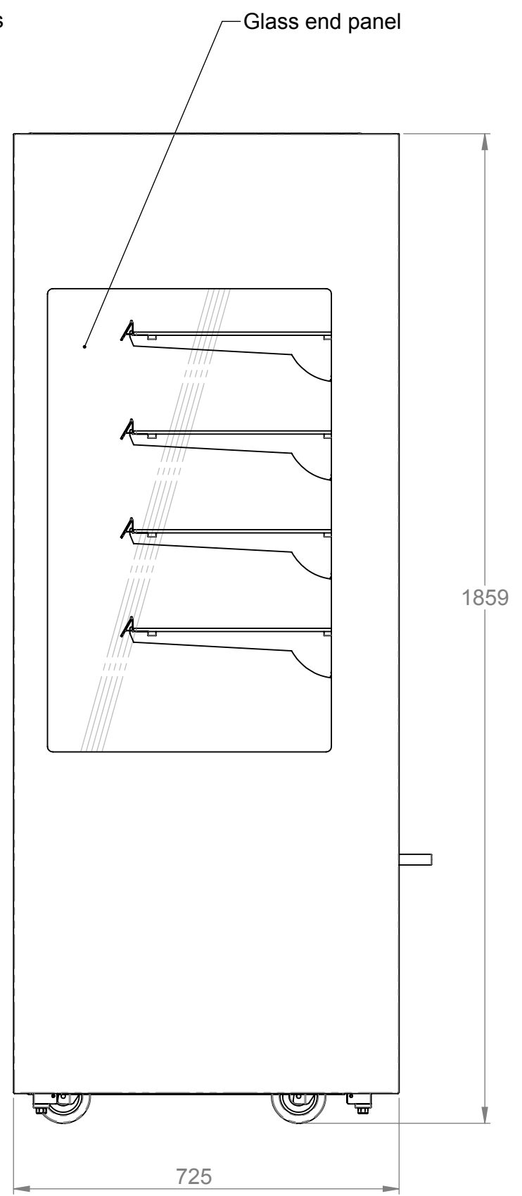
End elevation
