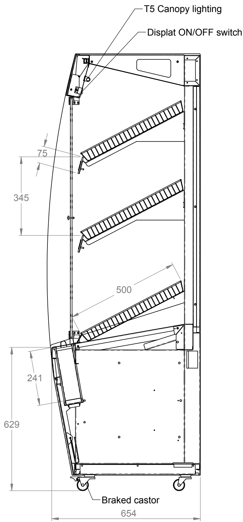
SECTION A-A
