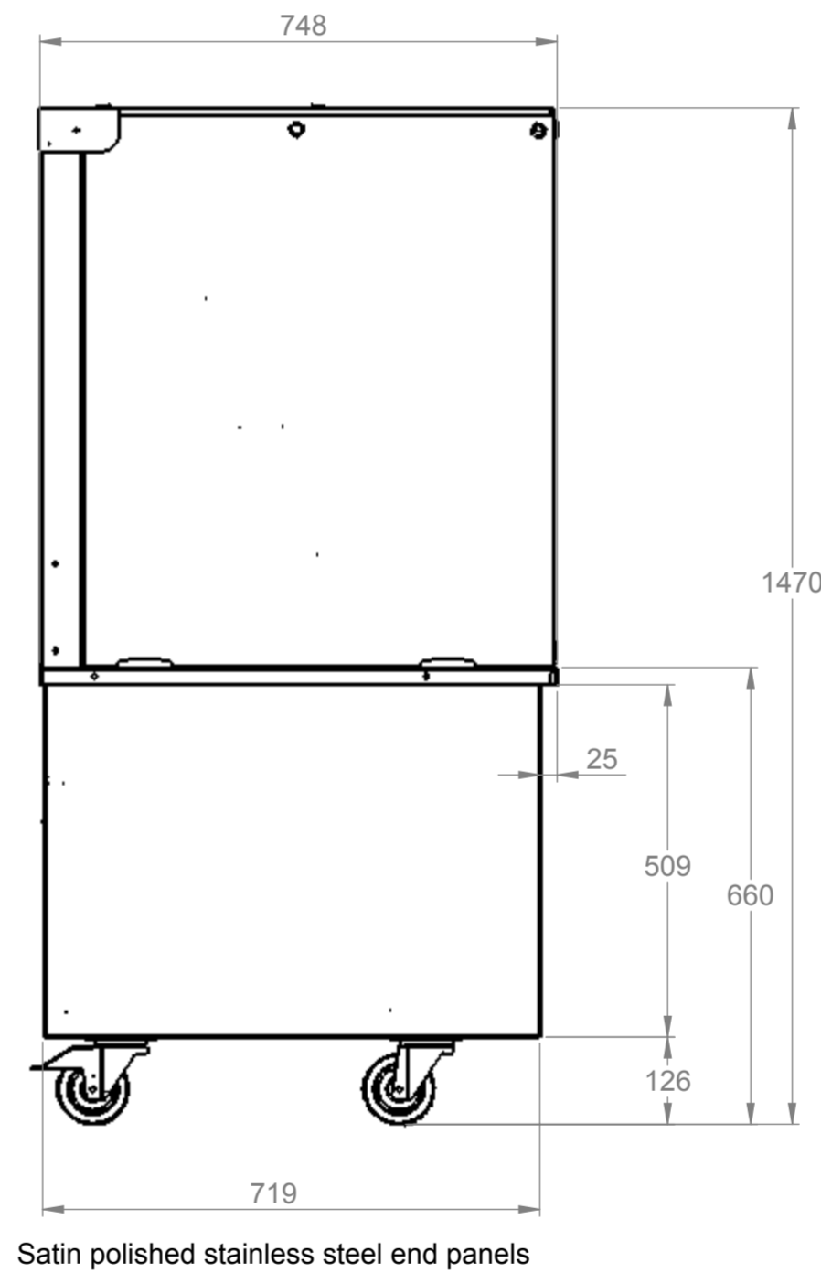
End elevation
