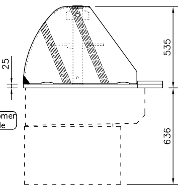
L.H. END ELEVATION
