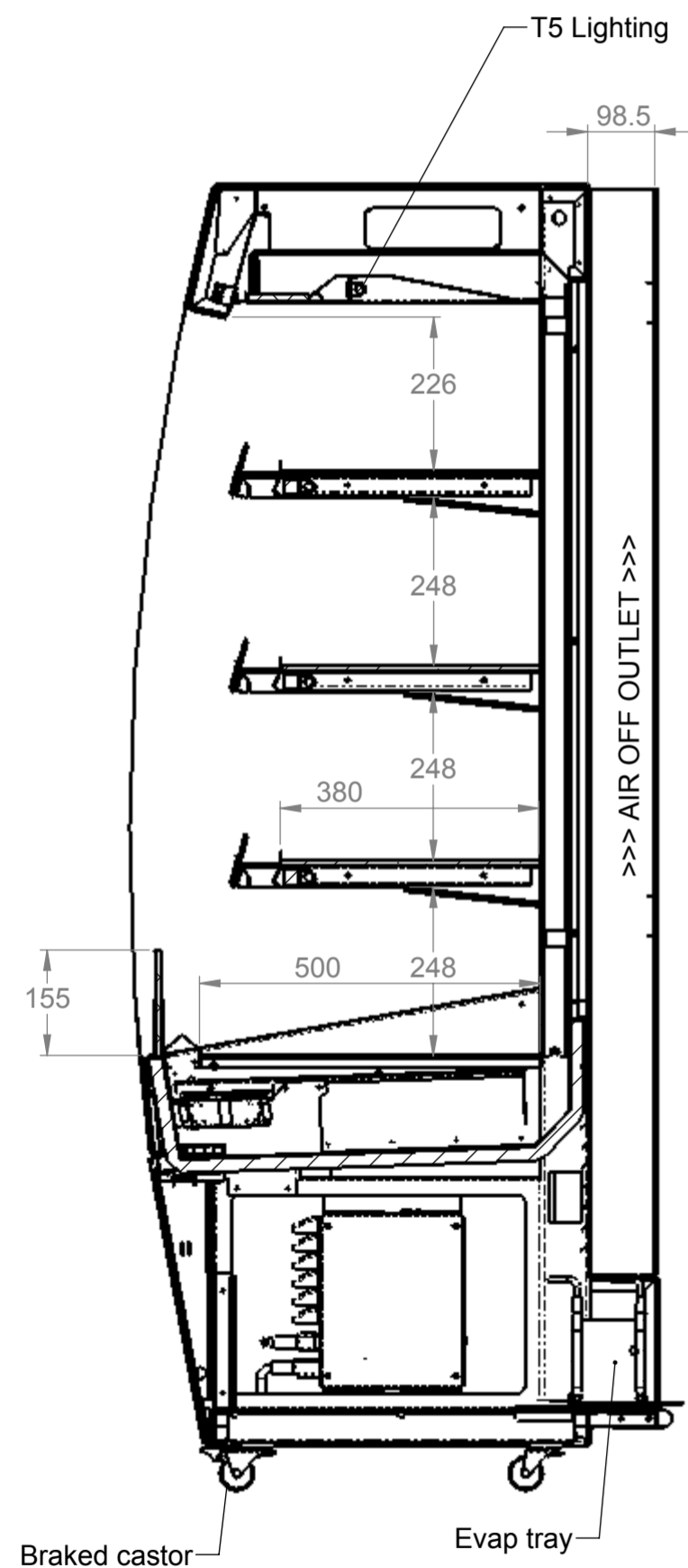
SECTION A-A
